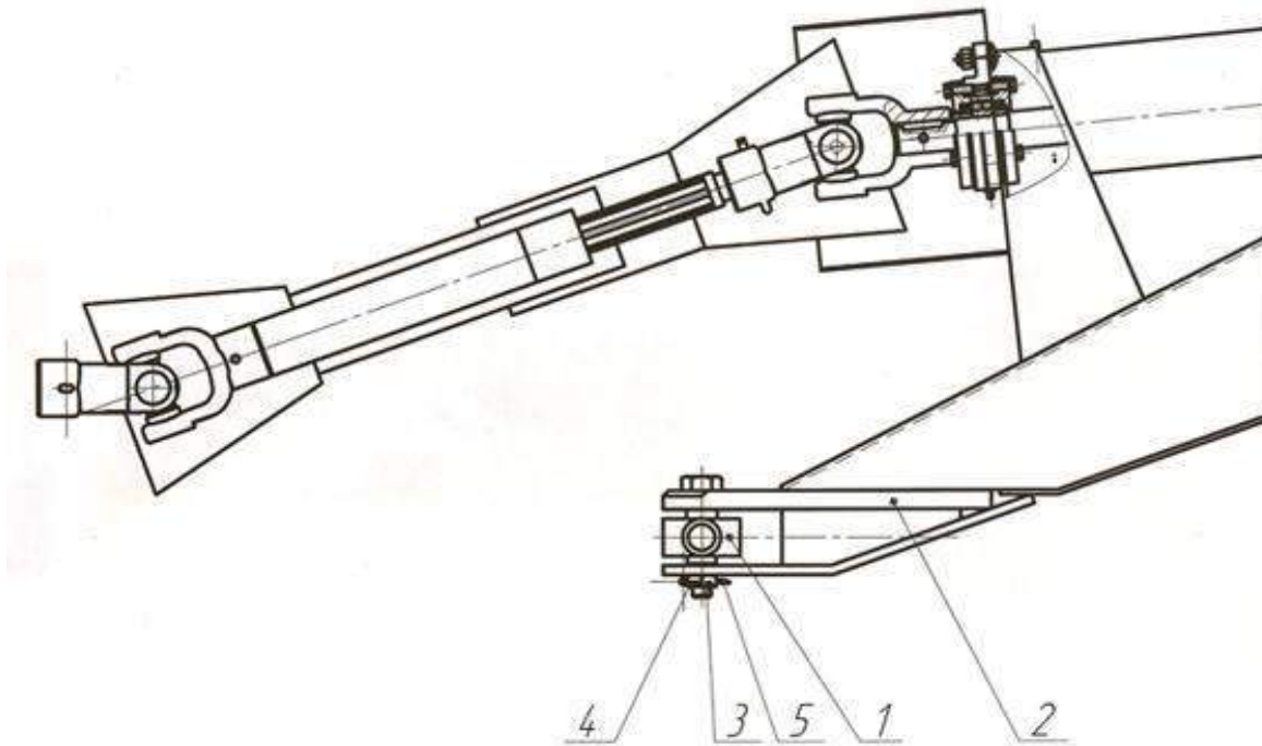
Рис. 2 Установка поперечной балки
